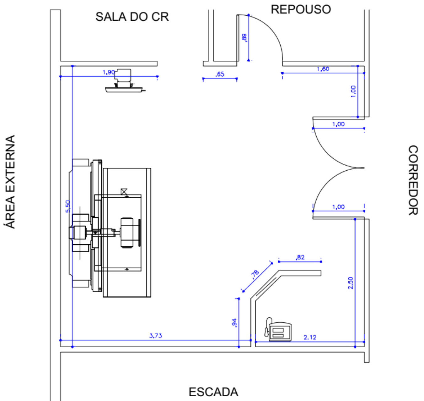
Figura 01. Planta com o equipamento de raios X
