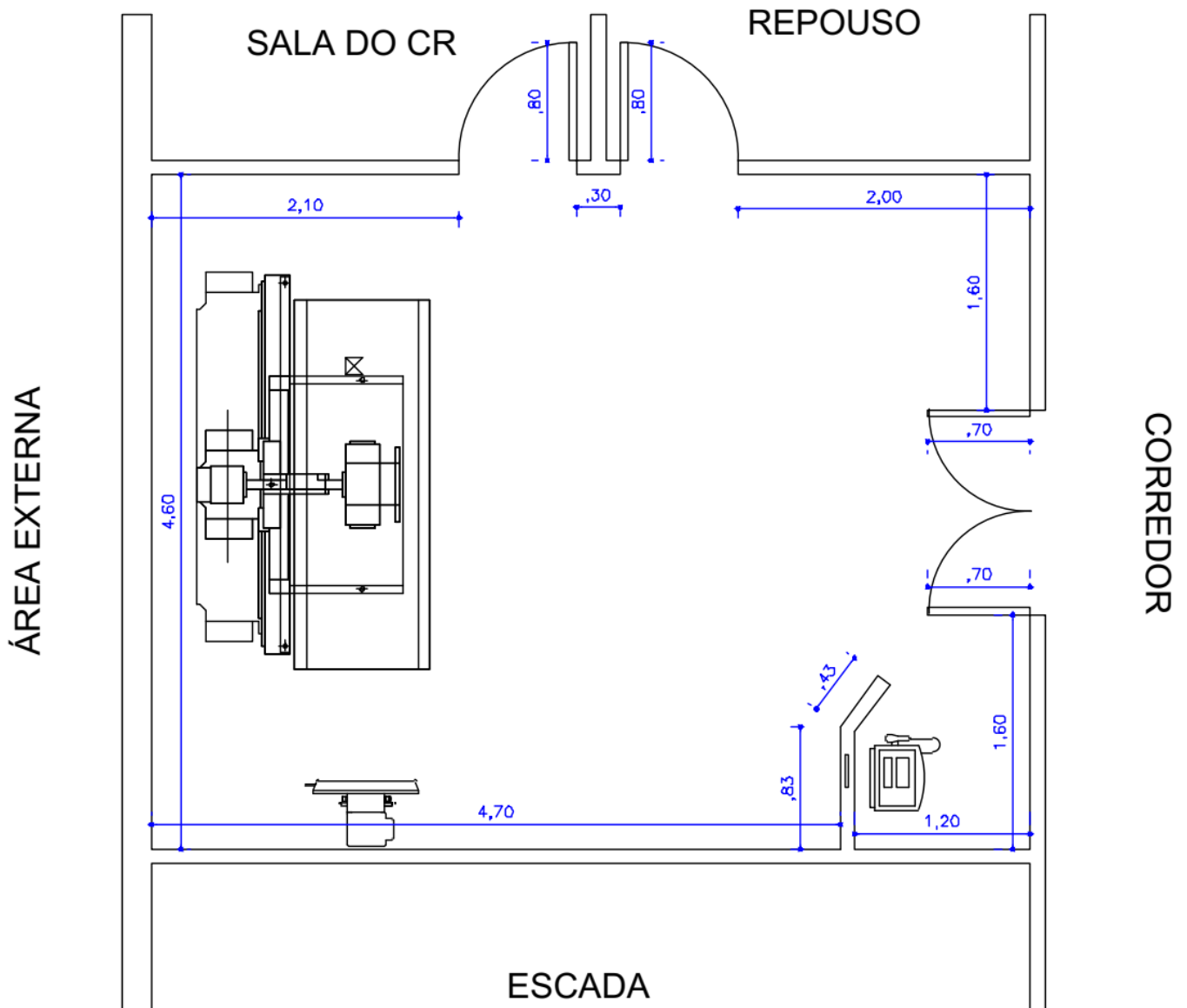
Figura 01. Planta com o equipamento de raios X
